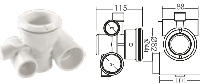
Ø32 Mm Hava ve Ø50 Su Çıkışlı Ø32 Mm Air and Ø50 Water Outlet
