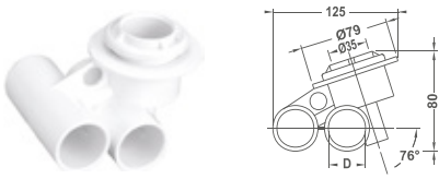
Ø32 Mm Hava ve Ø32 Su Çıkışı Ø32 Mm Air and Ø32 Water Outlet
