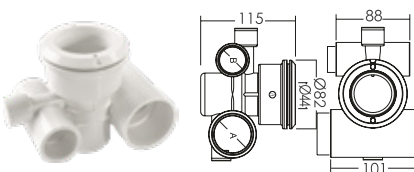
Ø32 Mm Hava ve Ø50 Su Çıkışlı Ø32 Mm Air and Ø50 Water Outlet
