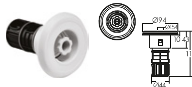
Düz Görünümlü (Standart) Jet Smooth Face (Swirl Jet)
