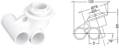
Ø32 Mm Hava ve Ø32 Su Çıkışlı Ø32 Mm Air and Ø32 Water Outlet
