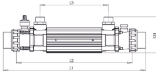
Elecro G2 Isı Eşanjörü Ebatları ΔT 30°C Rehberi Elecro G2 Heat Exchanger Sizing Guide for ΔT 30°C
